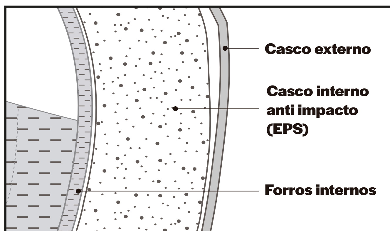
Seção da estrutura interna do capacete
