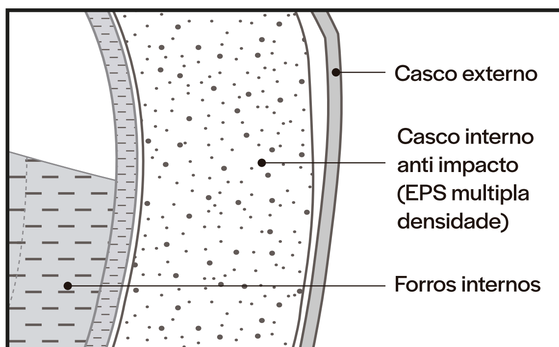
Seção da estrutura interna do capacete
